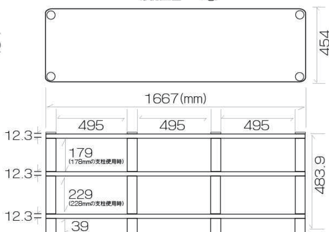
XWL03G寸法図 (製品重量 kg)
